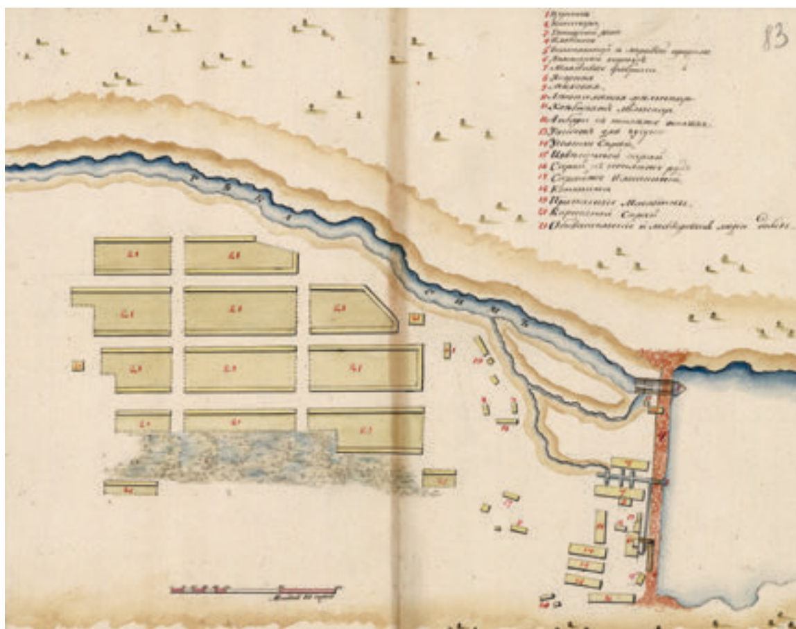
Симский железный завод [ГАСО. Ф. 101. ОП. 1. Д. 947. Л. 83 (план)]
