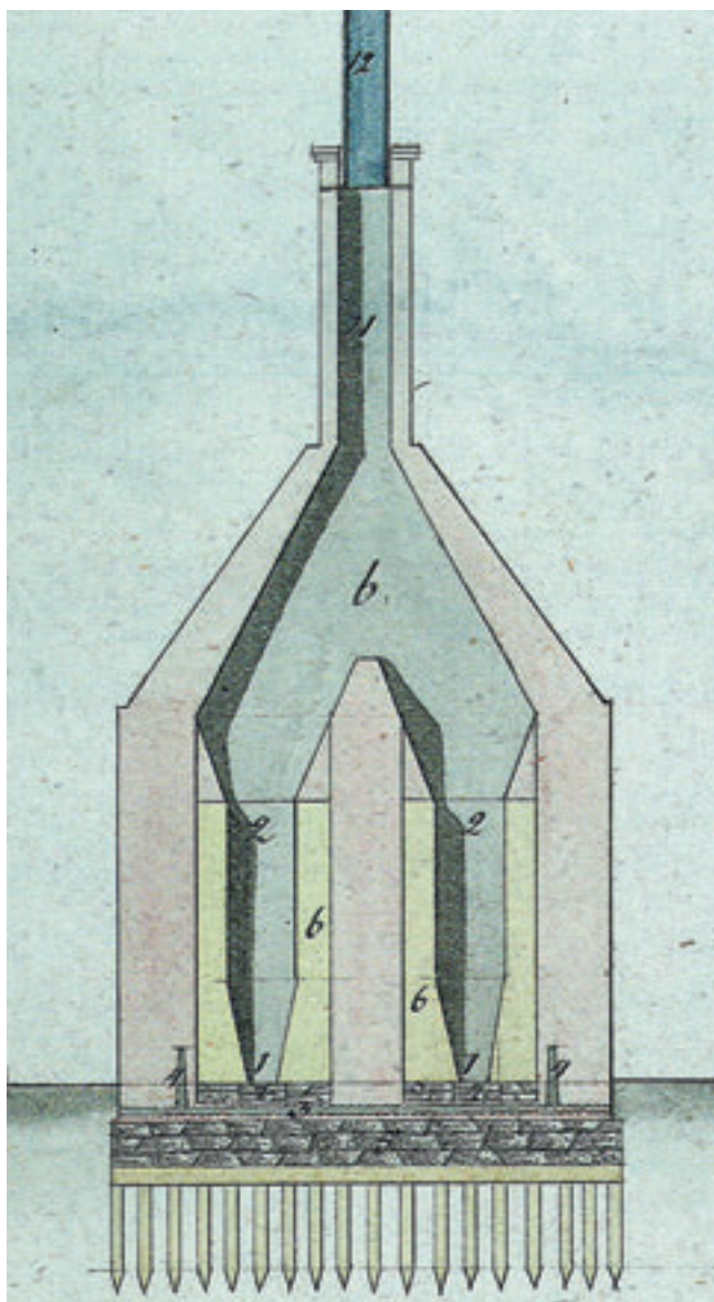
Медеплавильные печи Златоустовского завода. 1811 год.
