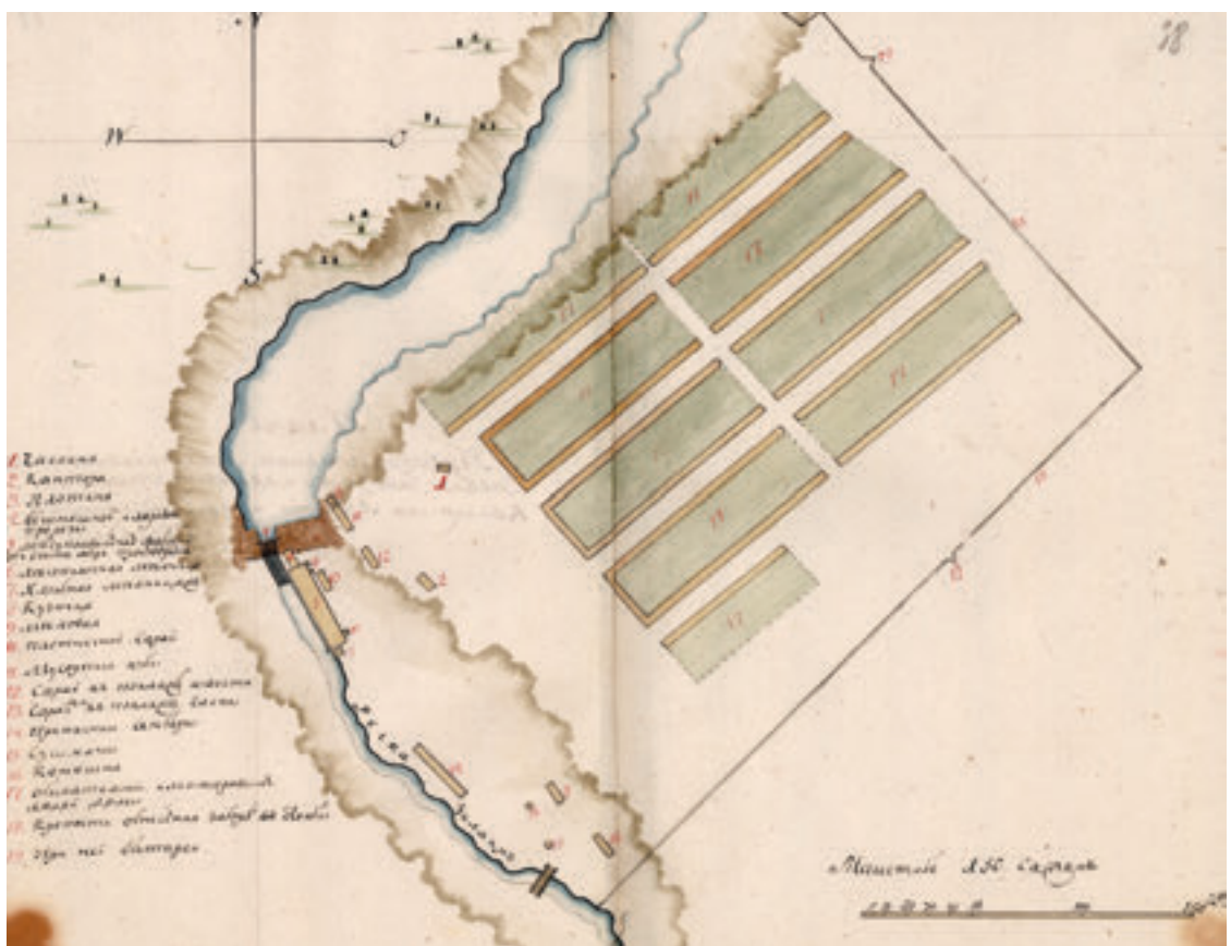
План Преображенский медеплавильный завод коллежского ассестора и заводосодержателя Твердышева. [ГАСО Ф. 101. ОП. 1. Д. 947. Л. 38]
