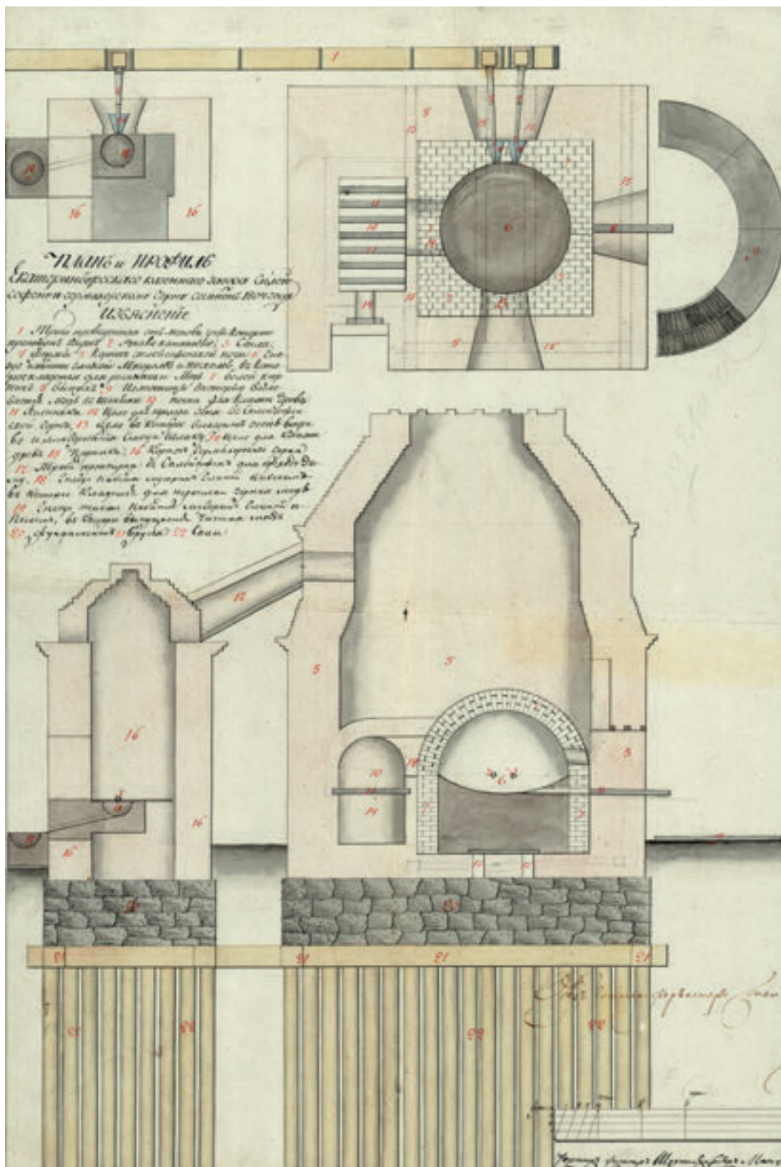
План и профиль сплейсофену и гармахерскому горну Екатеринбургского завода казенного 1804 года
