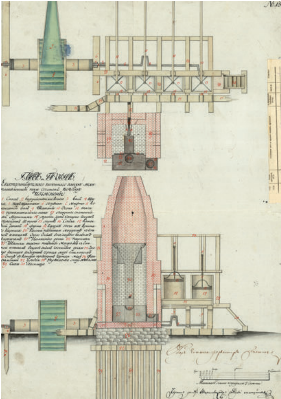
План и профиль медеплавильной печи 1804 года Екатеринбургского казенного завода. Изъяснения. 1. Спуск; 2. Вододействующее колесо; 3. Вал; 4. Шипы; 5. Подшипники; 6. Подушки; 7. Муфта; 8. Коленчатый вал; 9. Шатуны; 10. Очеп; 11. Тяги; 12. Призматические меха; 13. Патроны с кожаными поршнями; 14. Трубки, через которые воздух проходит в трубу; 15. Трубы; 16. Сопла; 17. Кожаный рукав; 18. Фурма; 19. Корпус печи из красного кирпича; 20. Колоша, набитая мусором, глиной и песком, около оных выложено белым кирпичом; 21. Наличные доски; 22. Парники; 23. Шестки, также набиты мусором с глиной и песком, вокруг оных чугунные доски; 24. Гнездо, в которое выходит черная медь со шлаком; 25. Гнездо, в которое проходит черная медь; 26. Фундамент; 27. Брусья; 28. Укрепления под мехами; 29. Сваи; 30. Лестница [ГАСО. Ф. 59. ОП. 7. Д. 346]
