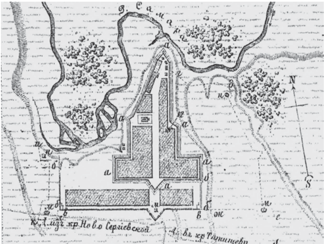
План Переволоцкой крепости [Ласковский Ф. «Карты, планы и чертежи к III части материалов для истории инженерного
