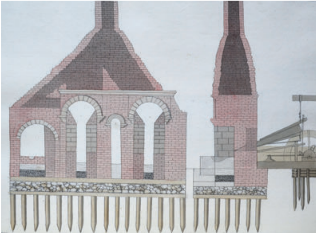
Широкий корпус (слева) гармахерского и сплейсофенного горнов. Корпус медеплавильной печи с клинчатыми мехами (справа) [Геннин В. (рукопись). Книга Сибирских горных заводов. Часть 2. Архив ЛОИИ. Ф. 115. ОП. 1. Д. 1161. Л. 74 75]
