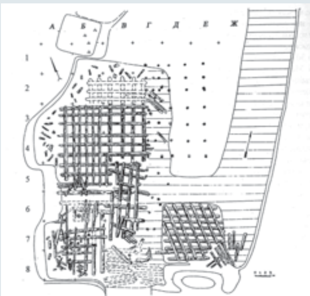
Свайно-реевое основание сливного моста
