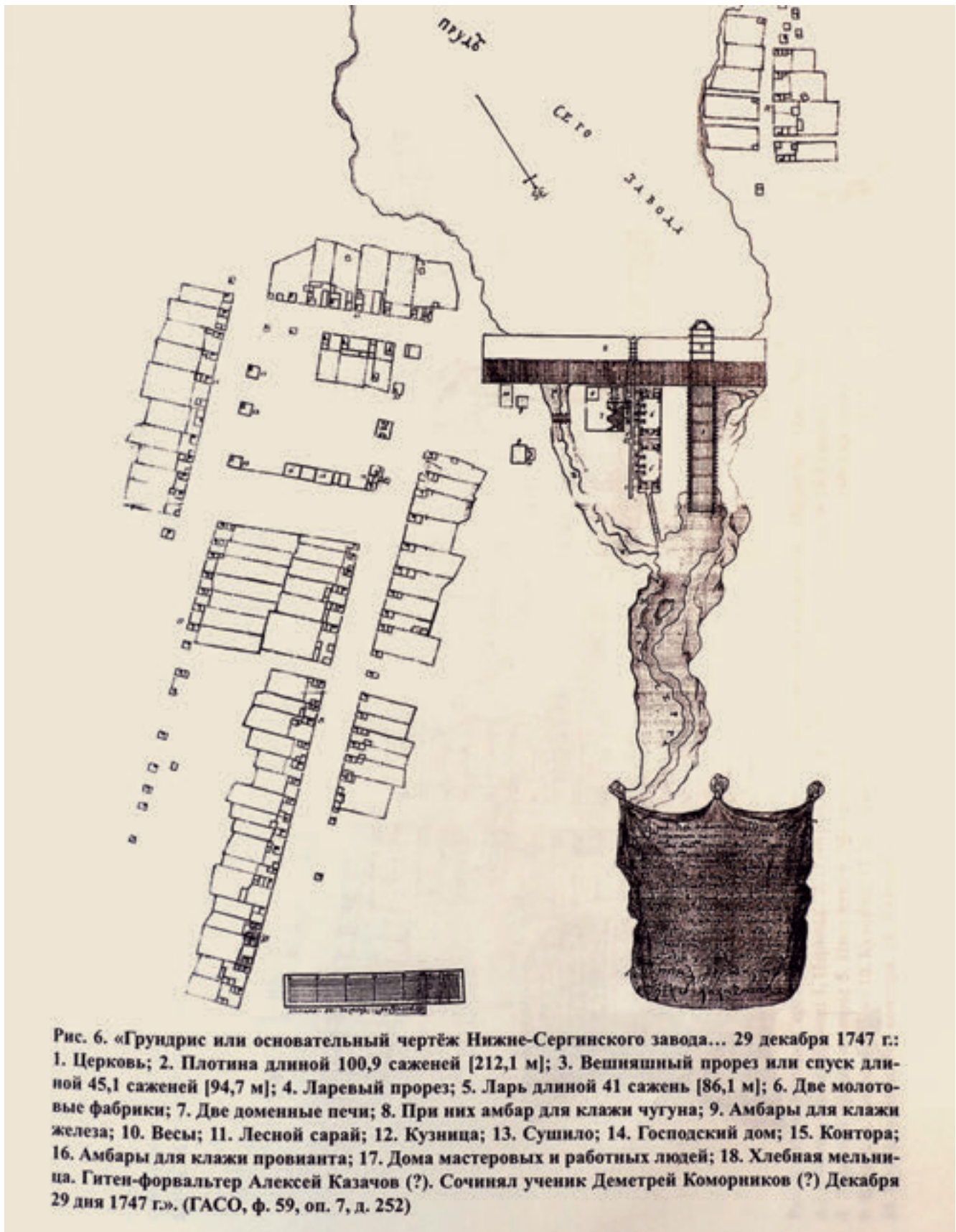
План Нижне-Сергинского завода [ГАСО. ф. 59. Оп. 7. Д. 252]
