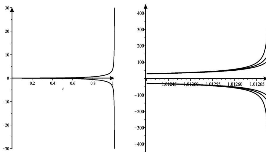
Рис. 2. Неустойчивость решения в окрестности точки нуль при \alpha = 5, \beta = 2, \lambda = 6, \lambda_0 = 5
