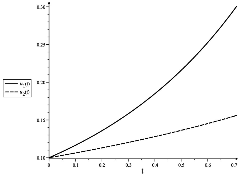
Рис. 1. Неустойчивость решения в окрестности точки нуль при \alpha = 3, \beta = 2, \lambda = 6, \lambda_0 = 5
