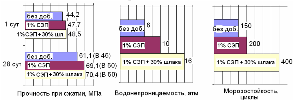
Рис. 13 – Характеристики бетонов после ТВО
