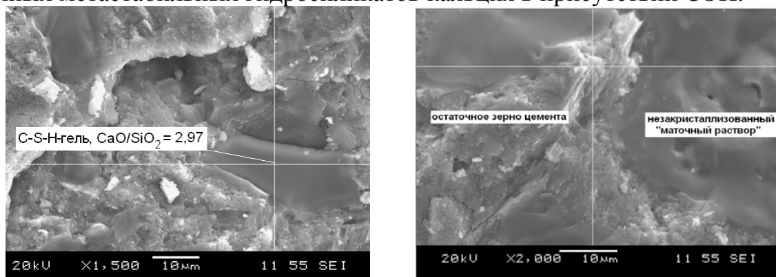
Рис. 5 – Структура цементного камня водного твердения с 1,2% СЭП
