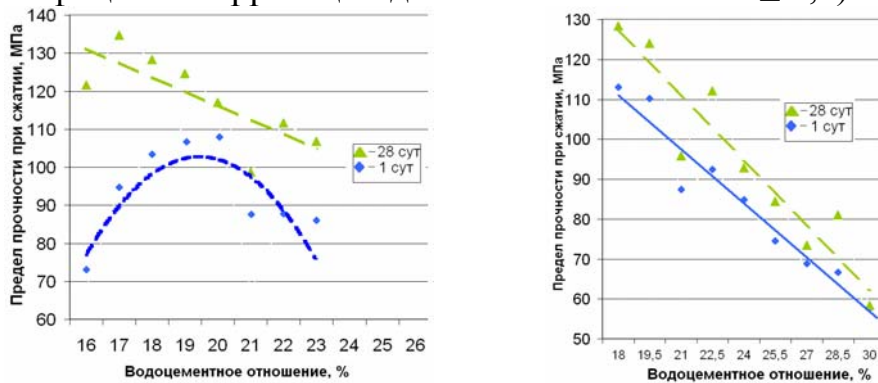
а) комплекс «СЭП + шлак» б) комплекс «СЭП + МТК» Рис. 3 – Зависимости прочности при сжатии цементного камня после проведения ТВО от водоцементного отношения
