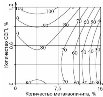
б) комплекс «СЭП + МТК»
