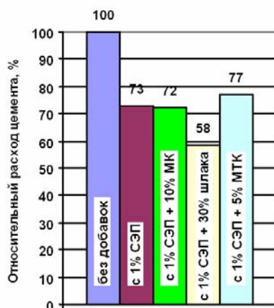
Рис. 10 – Относительный расход цемента в полученных бетонных смесях
