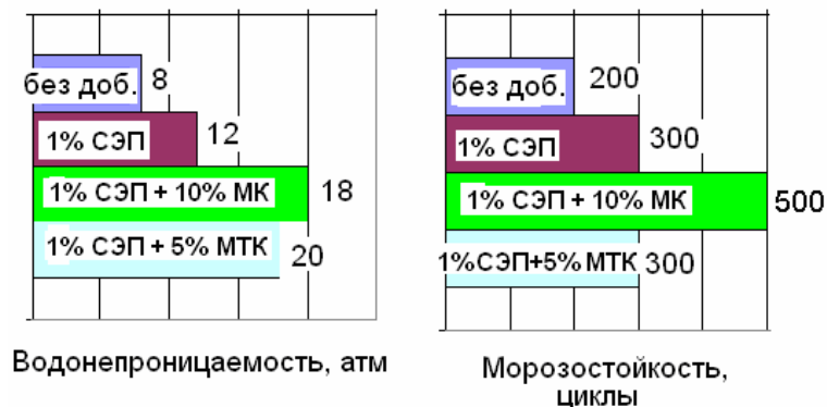
Рис. 12 – Свойства бетонов нормального твердения
