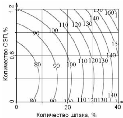
а) комплекс «СЭП + шлак»
