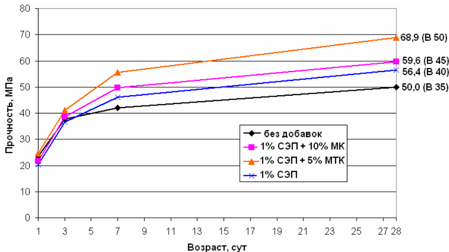
Рис. 11 – Прочность при сжатии бетонов нормального твердения
