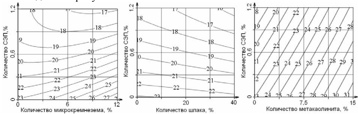
а) комплекс «СЭП + МК» б) комплекс «СЭП + шлак» в) комплекс «СЭП + МТК»
